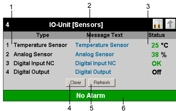
Abb. 32 Übersicht Sensoren an einer I/O-Unit
