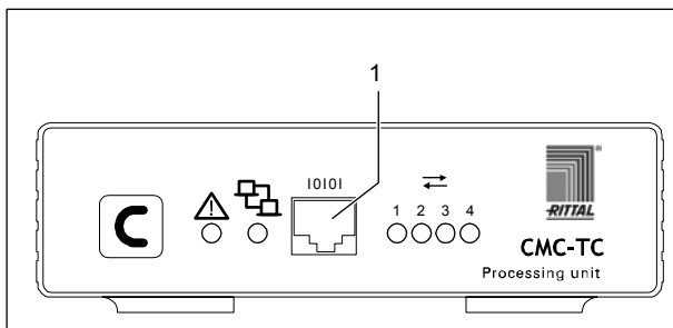
Abb. 15 RS-232-Anschluss
