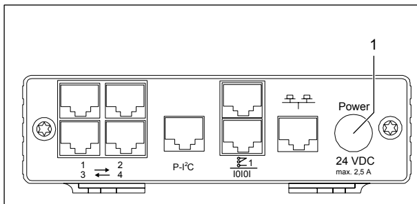
Abb. 6 Spannungsversorgung anschließen
