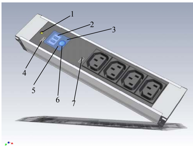
Abb. 34 ActivePSM (4-fach)
