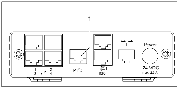
Abb. 14 P-I²C-Anschluss
