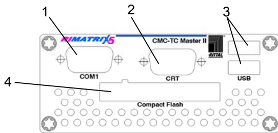
Abb. 1 CMC-TC Master II Vorderseite
