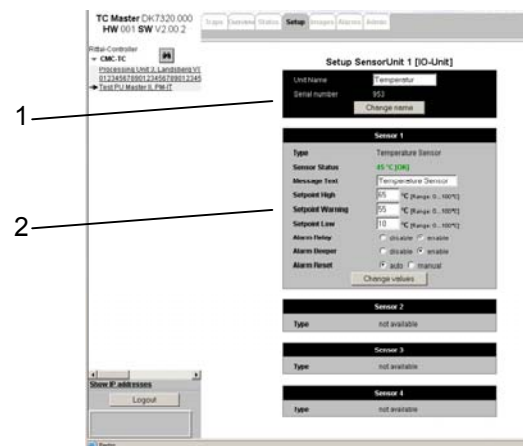
Abb. 38 Übersicht Einstellungen Sensoreinheiten
