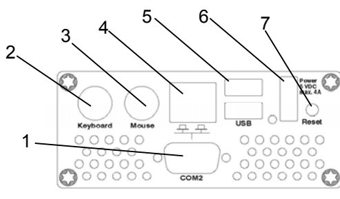
Abb. 2 CMC-TC Master II Rückseite
