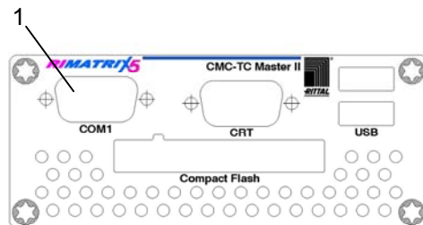
Abb. 8 RS-232-Anschluss
