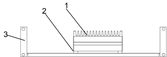
Abb. 4 Montage auf einen 2 HE Geräteboden
