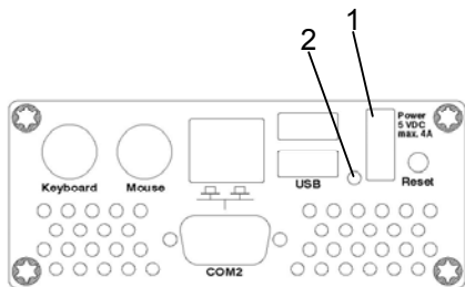
Abb. 6 CMC-TC Master II Spannungsanschluss
