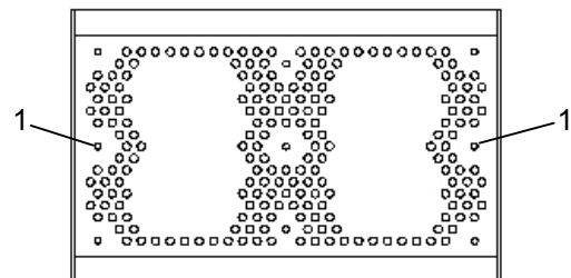
Abb. 5 Montage der Hutschienenhalter
